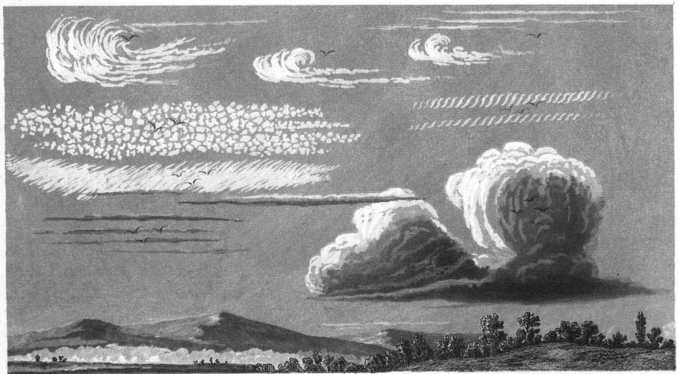
Cirrocumulus (Cir-Cum.)
